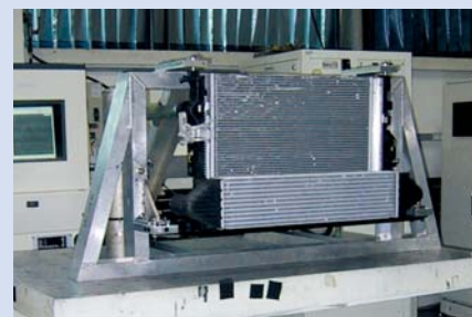
Testing engine cooling modules on a long-stroke shaker at Valeo Thermique Moteur, La Verrière/France
